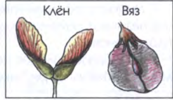
4.4. Плоды-крылатки.
