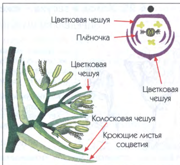
24.7. Колосок злака.
