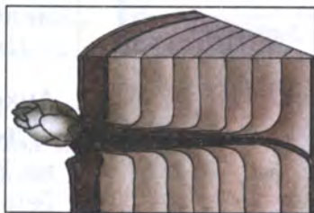
8.6. Пробудившаяся почка.
