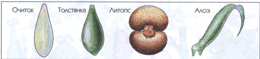
16.7. Мясистые листья.
