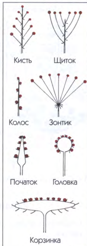
3.2. Схемы соцветий.
