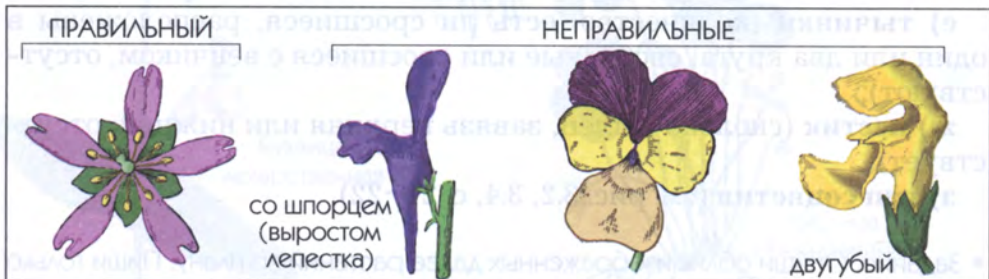
16.8. Цветки.
