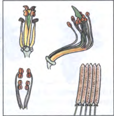
1.2. Многообразие тычинок.
